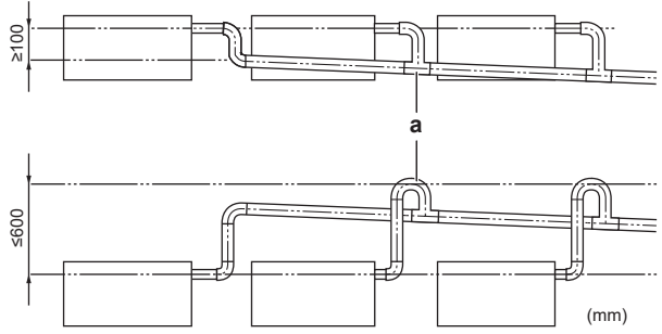
a T-bağlantı
