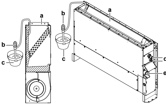
a Hava çıkışı b Taşınabilir pompa c Kova d Soğutucu boruları e Drenaj çıkışı
