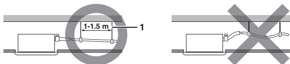
1 Závěsná tyč
