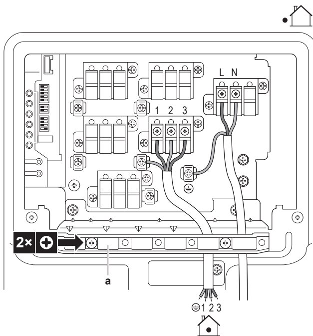
a Ledningsklemme
