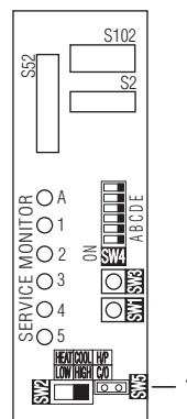
1 Schalter SW5 für Einstellung des Nachruhebetriebs
