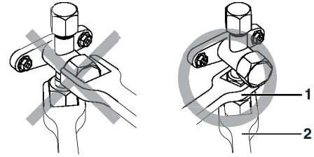
1 Moersleutel 2 Momentsleutel
