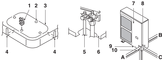
Εικόνα - Αγωγός εξωτερικού χώρου σε τέσσερις κατευθύνσεις
