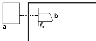
a Außeneinheit b Inneneinheit / Luftvorhang
