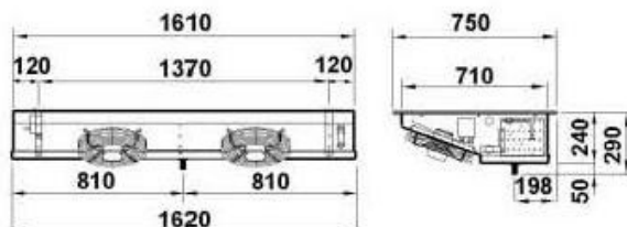
Evaporador GS340
