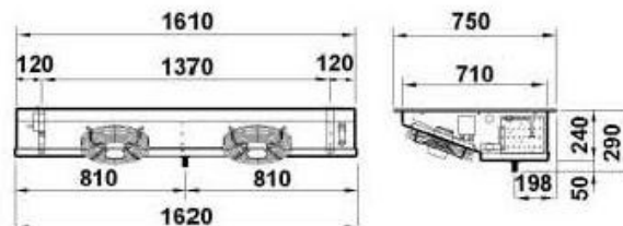
Verdampfer GS340
