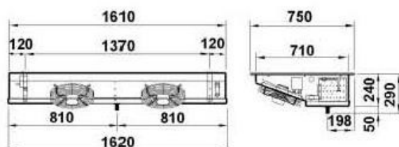
Evaporateur GS340
