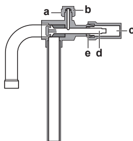
15-2 Skruventil til avstenging: tverrsnitt
