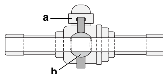
15-4 Kuleventil til avstenging: tverrsnitt
