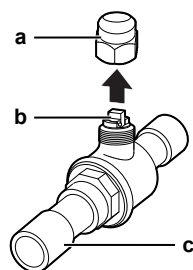
15-3 Kuleventil til avstenging: oversikt over komponenter
