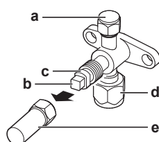
15-1 Skruventil til avstenging: oversikt over deler
