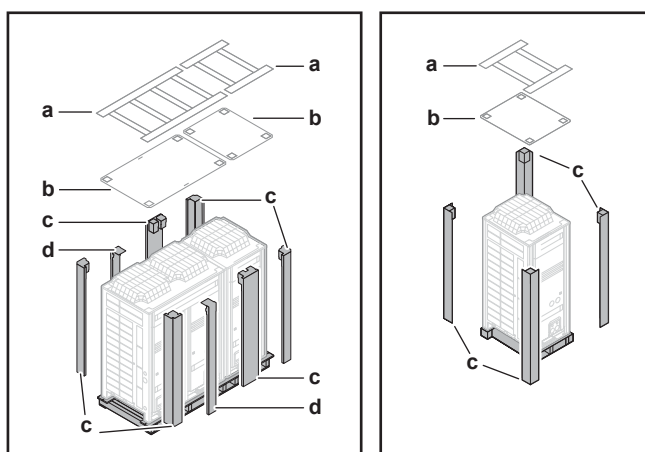
a Palette supérieure b Plateau supérieur c Cornière d Support intermédiaire (pour l'unité extérieure)
