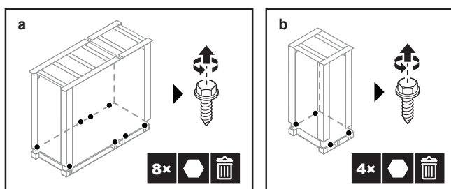
a Unité extérieure
