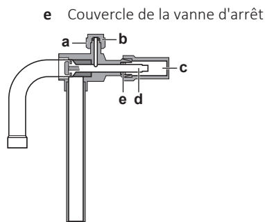
▲ 15-2 Vanne d'arrêt à vis: intersection
