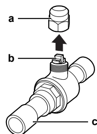
▲ 15-3 Vanne d'arrêt à bille: aperçu des pièces
