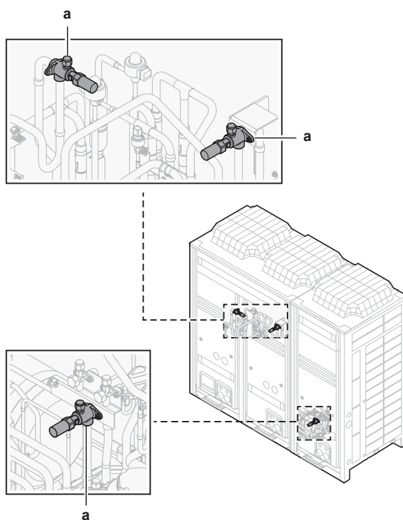
a Vanne d'arrêt pour maintenance
