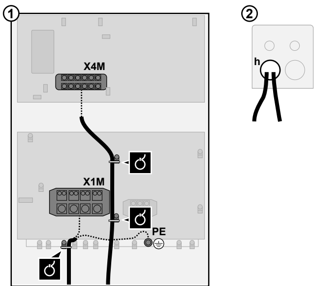
h Entrée de câblage (trou à enfoncer) pour haute tension. Voir "16.1.3 Directives pour la réalisation des trous à défoncer" [► 113].
