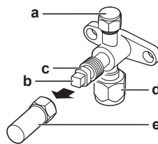
15-1 Válvula de cierre de tornillo: descripción de las piezas
