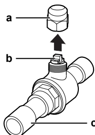
15-3 Válvula de cierre de bola: descripción de las piezas
