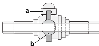
▲ 15-4 Válvula de cierre bola: intersección
