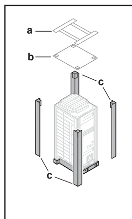
a Palé superior b Bandeja superior c Soporte angular d Soporte intermedio (para la unidad exterior)
