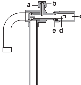
15-2 Válvula de cierre de tornillo: intersección
