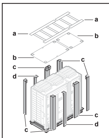
a Palé superior b Bandeja superior c Soporte angular d Soporte intermedio (para la unidad exterior)
