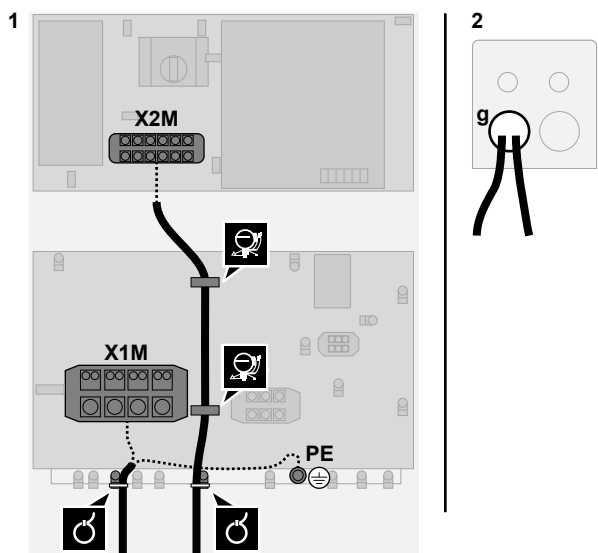
g Entrada del cableado (orificio ciego) para alta tensión. Consulte "16.1.3 Pautas para realizar orificios ciegos" [▶ 112].
