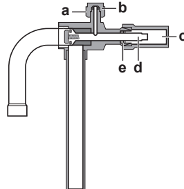
▲ 15-2 Βιδωτή βαλβίδα διακοπής: διασταύρωση
