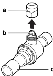
▲ 15-3 Σφαιρική βαλβίδα διακοπής: επισκόπηση εξαρτημάτων
