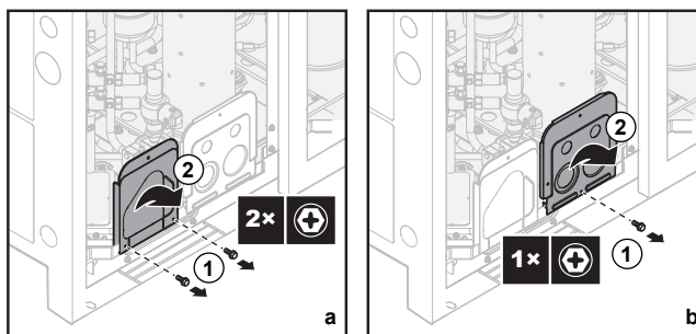
a (εάν εφαρμόζεται) Μικρή μπροστινή πλάκα αριστερά b Μικρή μπροστινή πλάκα δεξιά
