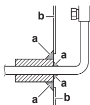
a Tætningsmateriale b Frontpanel
