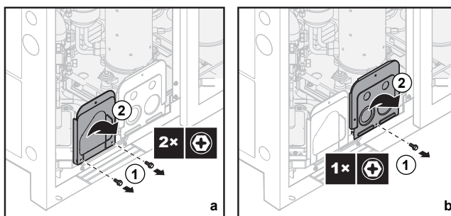
a (Hvis relevant) Lille frontplade venstre b Lille frontplade højre
