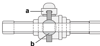
15-2 Kuglespærreventil: tværsnit
