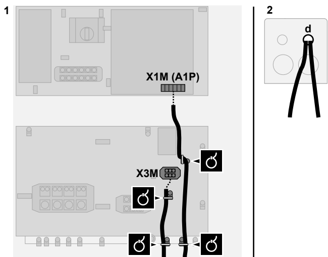
d Indføring af lavspændingsledninger (udstansningshul). Se "16.3 Åbning af forberedte huller" [▶ 112].
