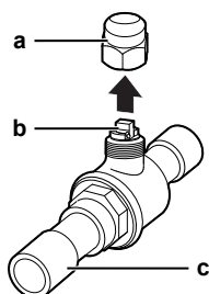
15-1 Kuglespærreventil: overblik over dele
