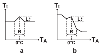
a TAI dorită absolută b TAI dorită - curbă în funcție de vreme
