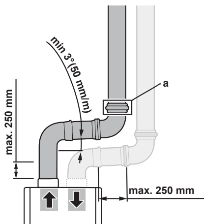
a Al doilea element după primul cot
