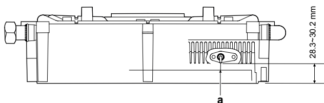
a Distanță scântei (±4,5 mm)
