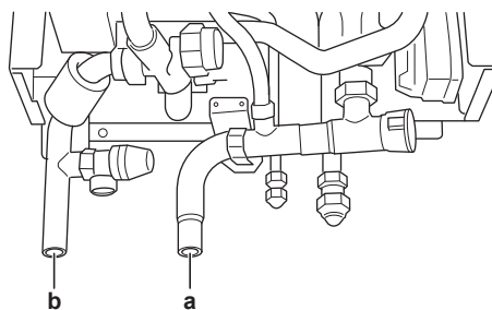
a Wassereinlass b Wasserauslass
