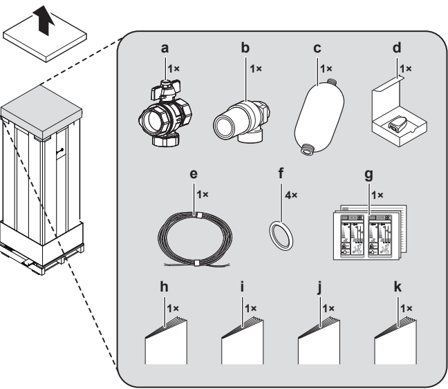
a Válvula de aislamiento con filtro integrado
