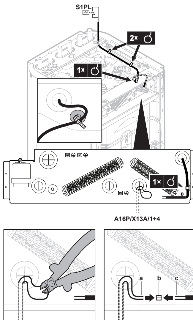
a Durchschnittene Kabelwindung von A16P/X13A/1+4 (werkseitig befestigt)
