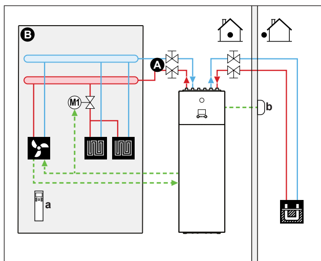
Схема
