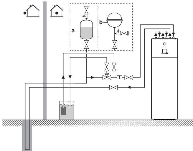
a Съд за контрол на нивото на соления разтвор (аксесоар) b Разширителен съд (доставка на място, ако съдът за солени разтвори не може да бъде монтиран в най-високата точка)
