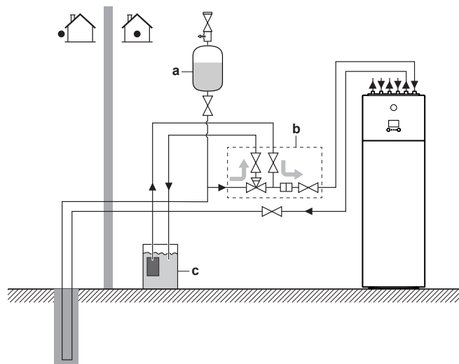
a Съд за контрол на нивото на соления разтвор (аксесоар) b Комплект за пълнене на солени разтвори (доставка на място или допълнителен комплект KGSFILL2) c Система за пълнене на солени разтвори (доставка на място)
