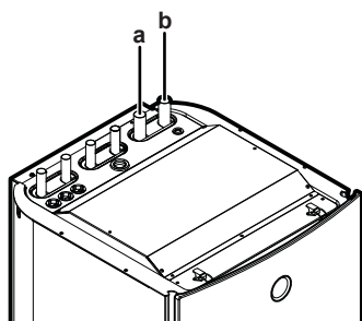
a ИЗХОДНО съединение за солени разтвор (Ø28 mm) b ВХОДНО съединение за солени разтвор (Ø28 mm)
