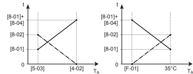
[8-04]: Дополнительный таймер при [4-02]/[F-01]
