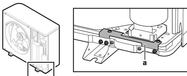
a Транспортировочная опора
