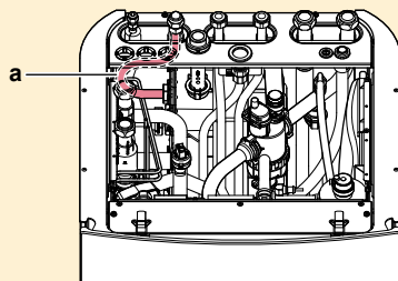
a Kjølemiddelgassrør
