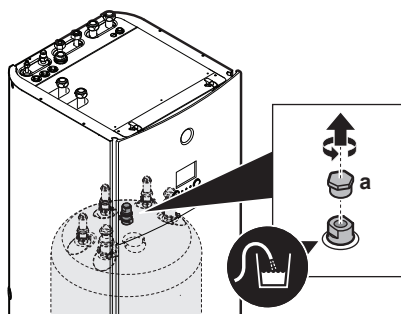
a Tartálynyílás
