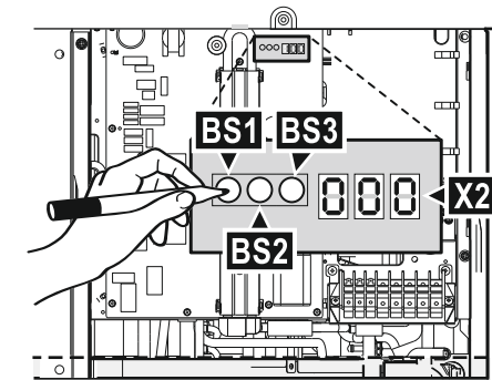
Écran à 7 segments
