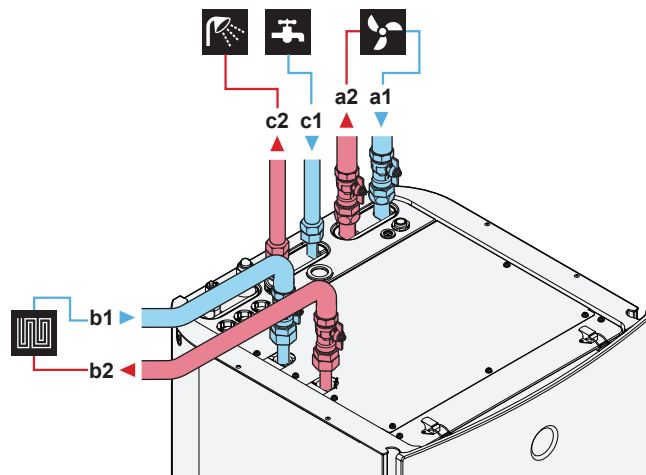
a1 Lisäalue – tilanlämmityksen/jäähdytyksen veden TULO (ruuviliitäntä, 1")
