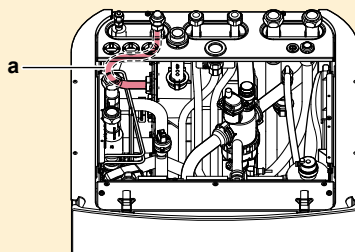
a Tubo de gas refrigerante
