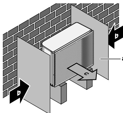
a Ablenkplatte
