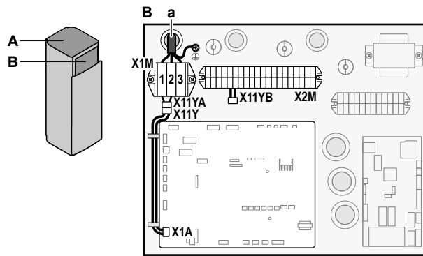
а Съединителен кабел (=главно електрозахранване)
