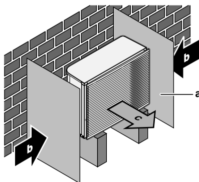
a Ветрозащитна преграда
