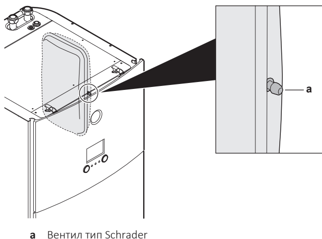
a Вентил тип Schrader
