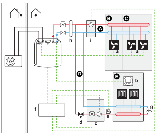
3 Sistem s hidravličnim ločevalnikom za obe območji: Pri tem sistemu je za dodatno območje potrebna neposredna črpalka.
