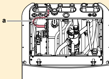
a Koelmiddelgasleiding
