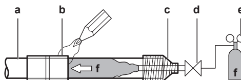
a Köldmediumrör
