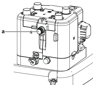
a Övertrycksventil
