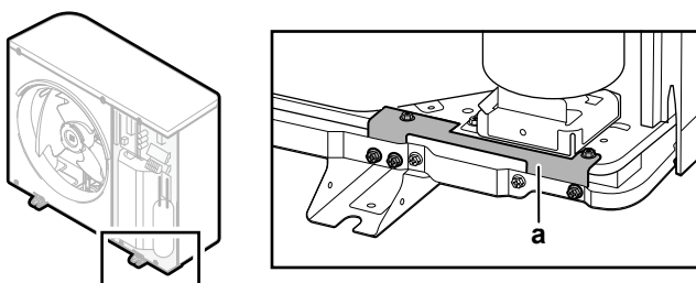
a Pritrdila za transport
