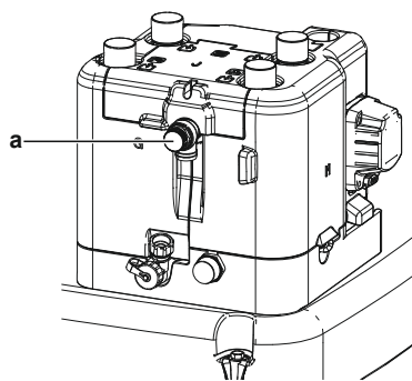
a Varnostni tlačni ventil
