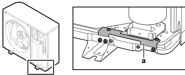
a Transportsicherung
