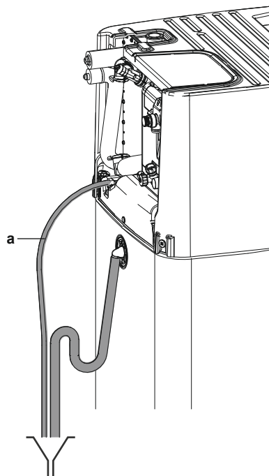
a Ablaufwannenschlauch
