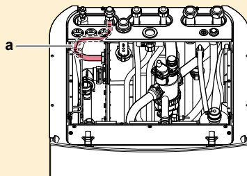
a Трубопровод газообразного хладагента
