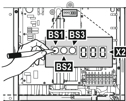
7-сегментный дисплей
