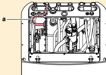
a Тръба за газообразен хладилен агент
