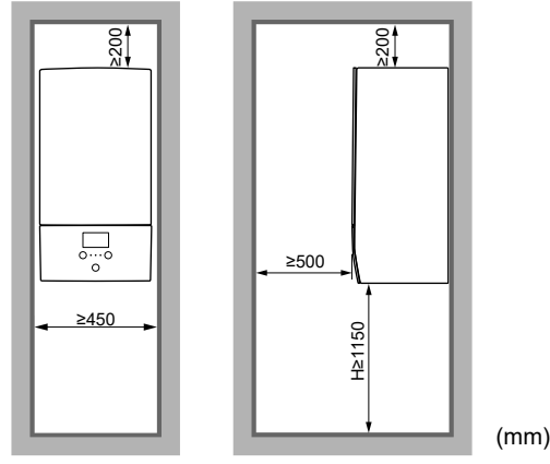
H Gövdenin altından zemine ölçülen yükseklik
