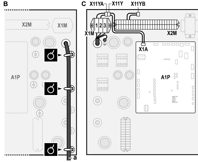
a Ara bağlantı kablosu (=ana güç kaynağı)
