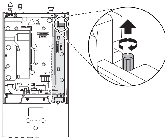
a Schraeder ventil
