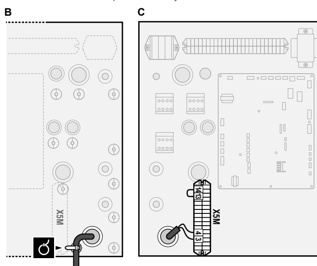
S4S Smart Grid impulsu skaitītājs
