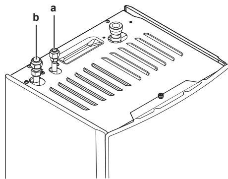
a Raccord du liquide réfrigérant b Raccord du gaz réfrigérant
