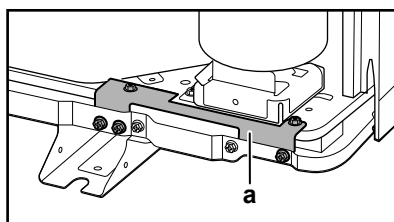
a Podpórka transportowa
