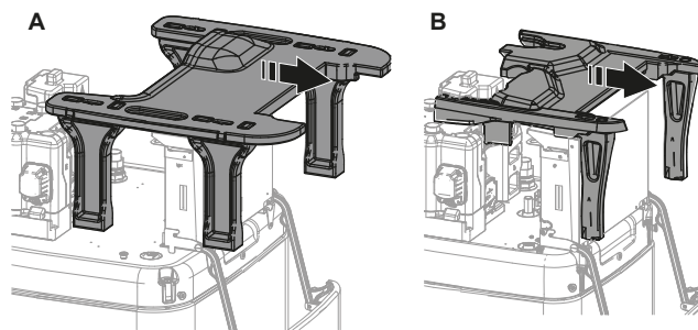
A За модели с резервоар за съхранение 500 l B За модели с резервоар за съхранение 300 l
