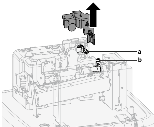
a, b Ръчен вентил на отворите за излизане на въздуха
