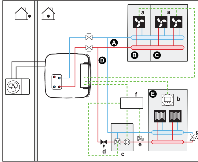
2 Ana bölge için hidrolik separatörlü sistem:
