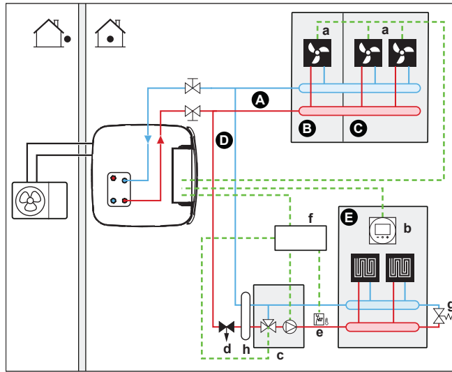
3 Her iki bölge için hidrolik separatörlü sistem:
