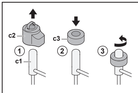
c1 Elektronický expanzný ventil
