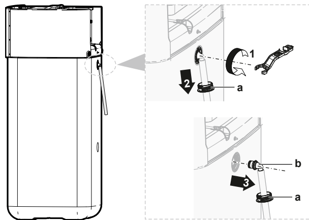
a Overloopaansluiting b Schroefplug
