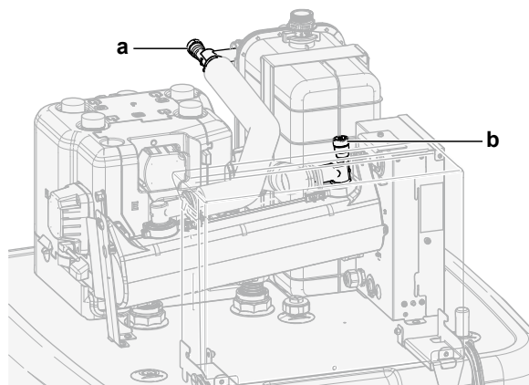
a, b Handbediende ontluichtingsklep
