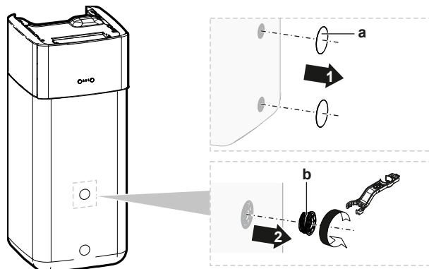
a Aansluitdeksel b Schroefplug
