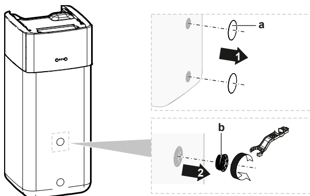
a Kryt připojení b Šroubová zátka
