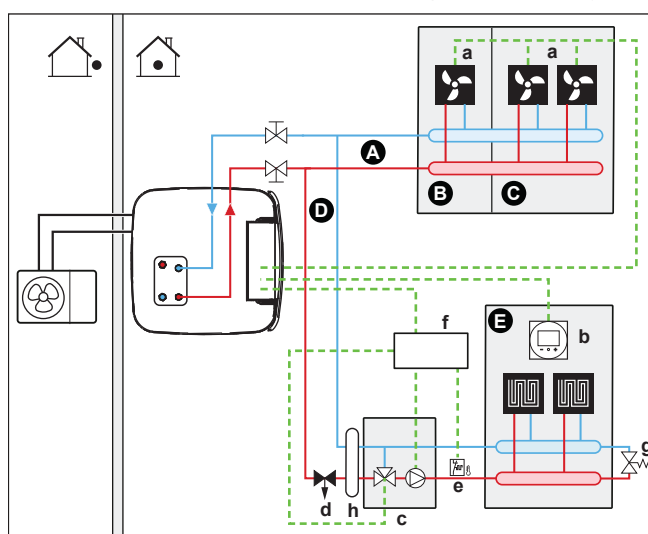
3 Sistem s hidravličnim ločevalnikom za obe območji: Pri tem sistemu je za dodatno območje potrebna neposredna črpalčka.
