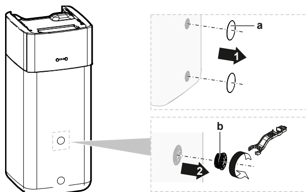
a Pokrov priključka b Navojni čep
