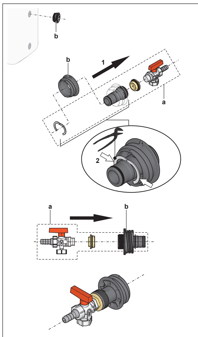
a Komplet za polnjenje in praznjenje b Navojni čep
