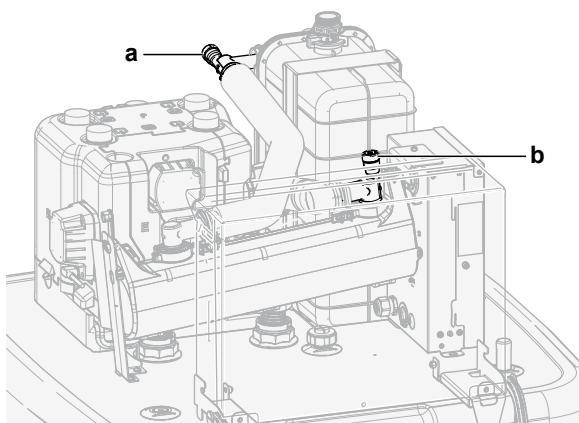
a, b Válvula de purga de ar manual
