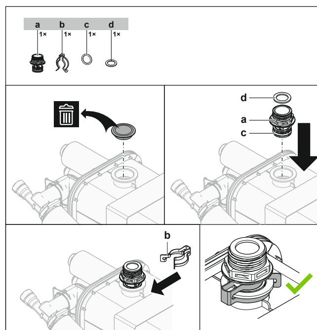
a Tomada da chaminé
