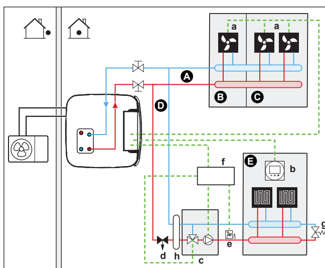
3 Sistema com separador hidráulico para ambas as zonas: Para este sistema, é necessária uma bomba direta para a zona adicional.
