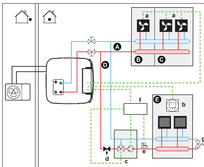
2 Sistema com separador hidráulico para a zona principal:
