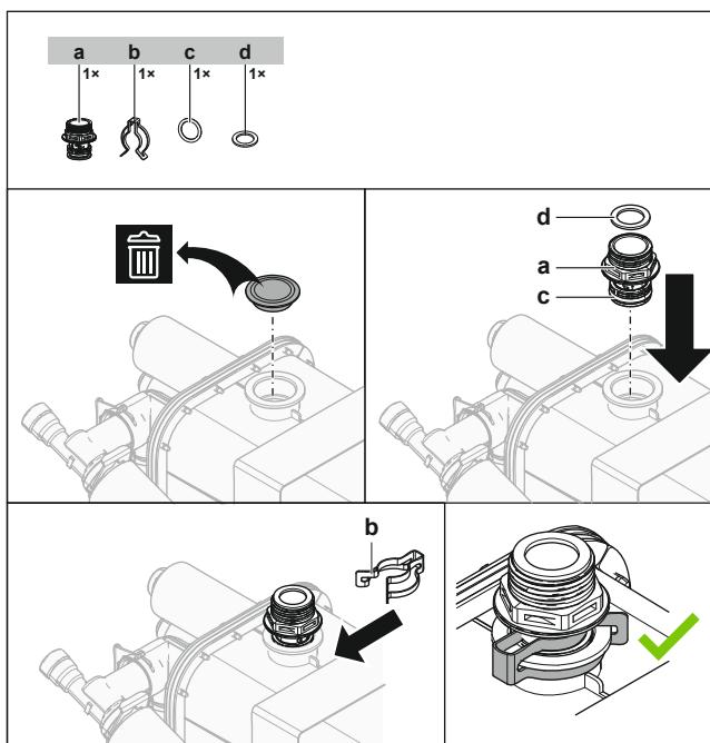
a Skorstensmuffe
