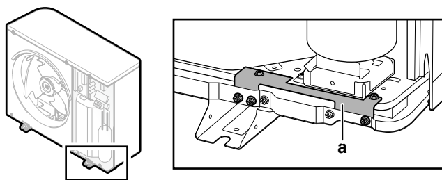
a Транспортировочная опора
