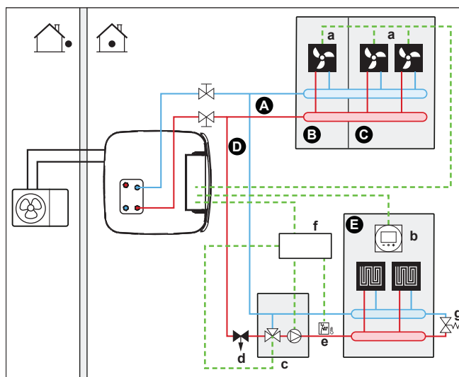
2 Sistema con separatore idraulico per la zona principale:
