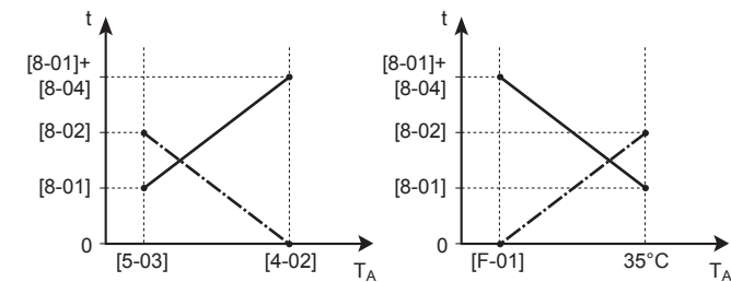
[8-04]: Timer aggiuntivo a [4-02]/[F-01]
