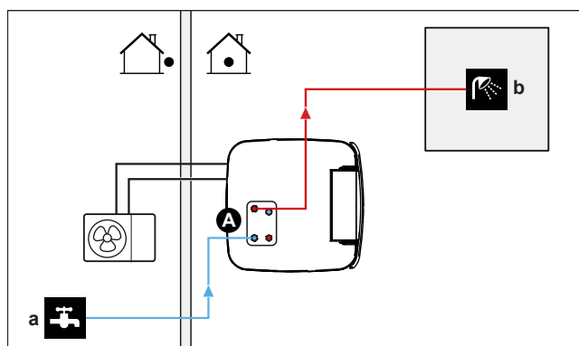
A Acqua calda sanitaria a Acqua fredda ENTRATA
