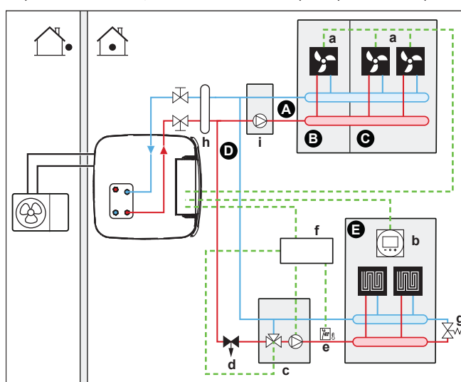
3 Sistema con separatore idraulico per entrambe le zone: Per questo sistema, è necessaria una pompa diretta per la zona aggiuntiva.
