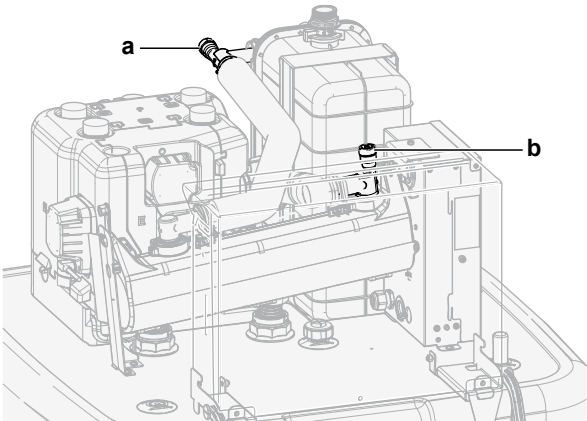
a, b Valvola di sfiato dell'aria manuale
