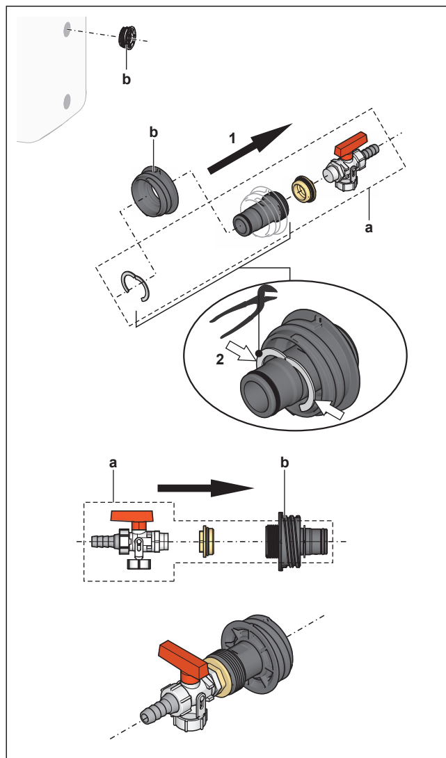
a Κιτ πλήρωσης και αποστράγγισης b Βιδωτό πώμα
