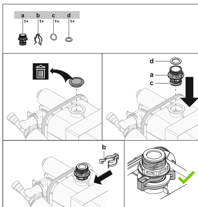
a Skorstensmuffe
